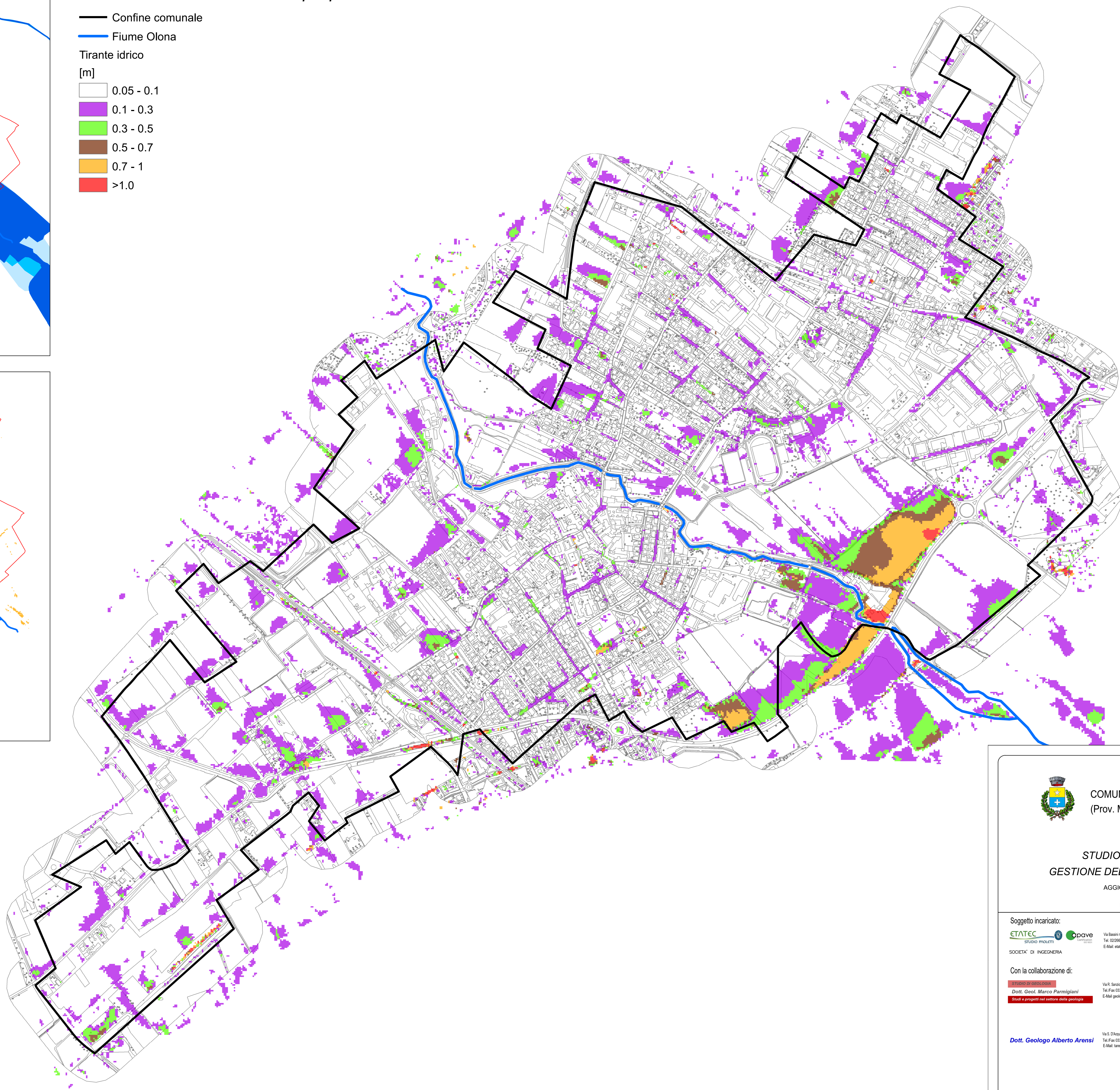
Portata T=10 anni Olona assetto attuale e precipitazione T=10 anni
