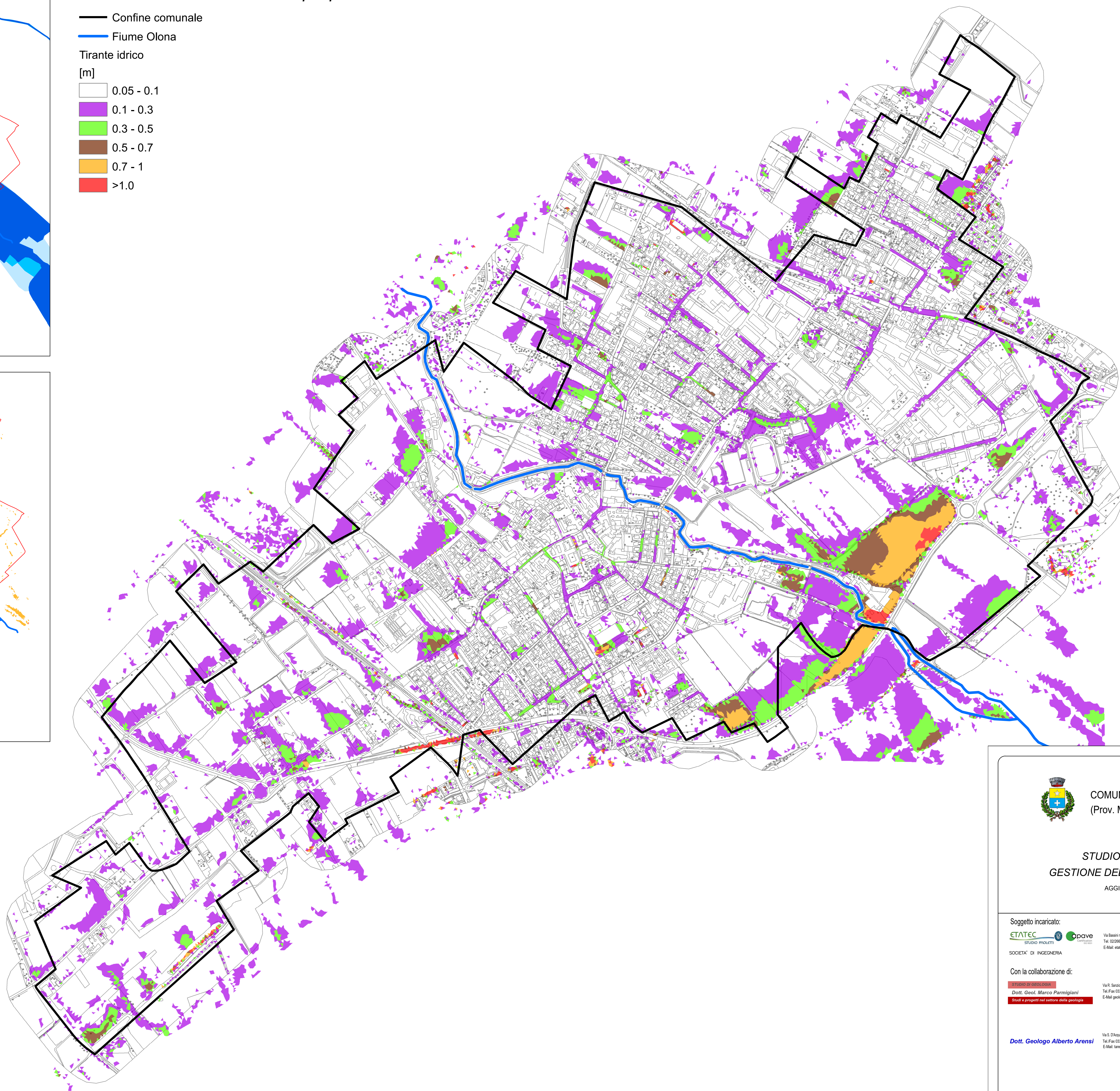
Portata T=10 anni Olona assetto attuale e precipitazione T=50 anni
