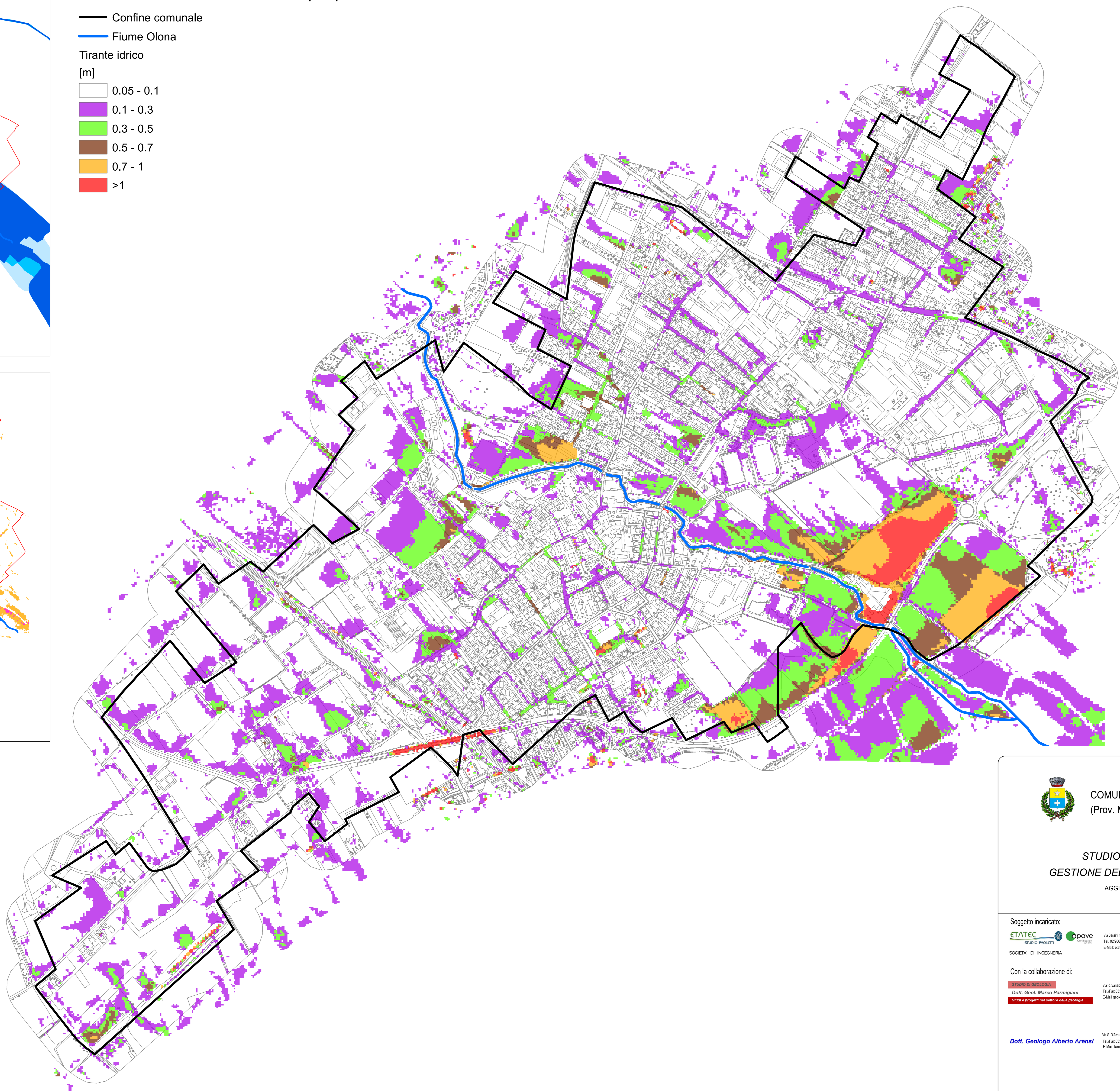
Portata T=100 anni Olona assetto attuale e precipitazione T=100 anni
