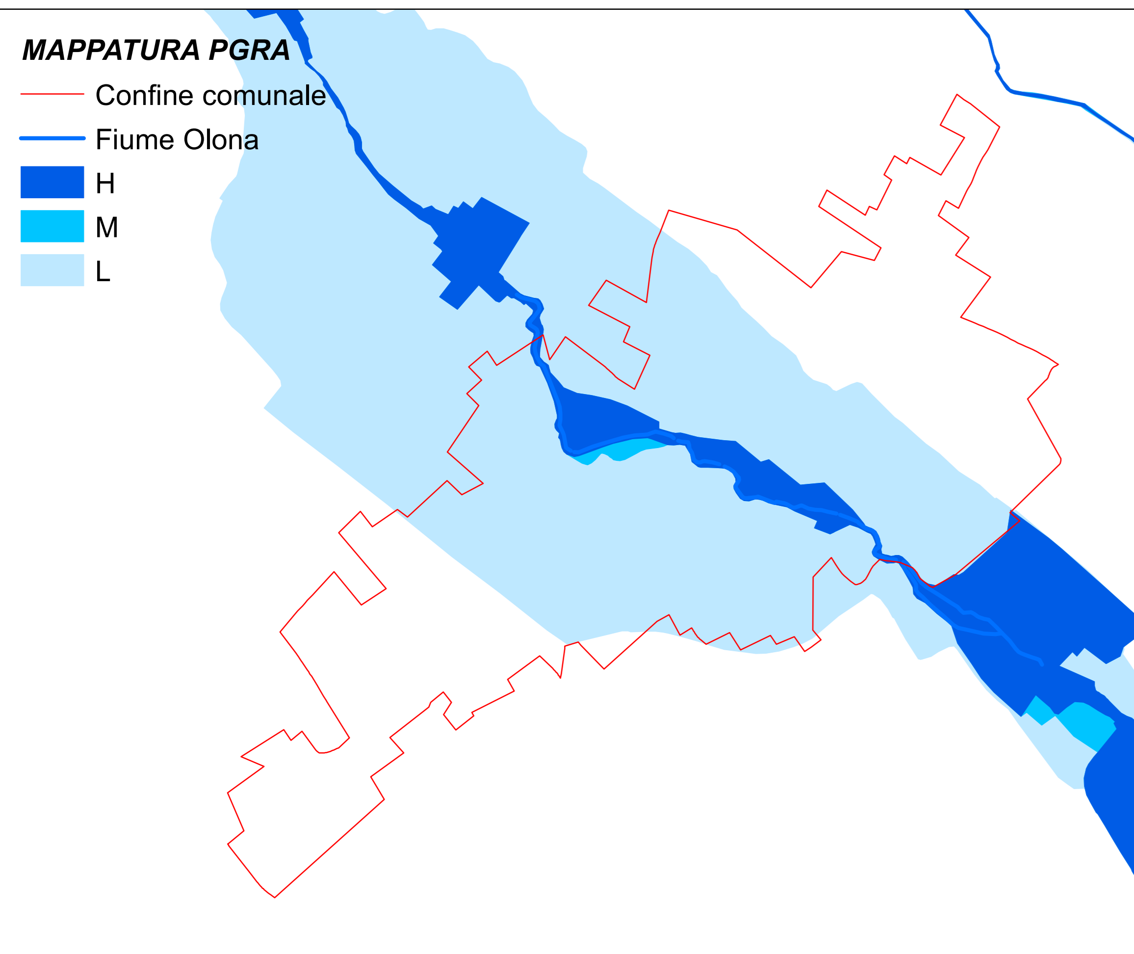
Portata di progetto T=100 anni Olona e precipitazione T=100 anni
