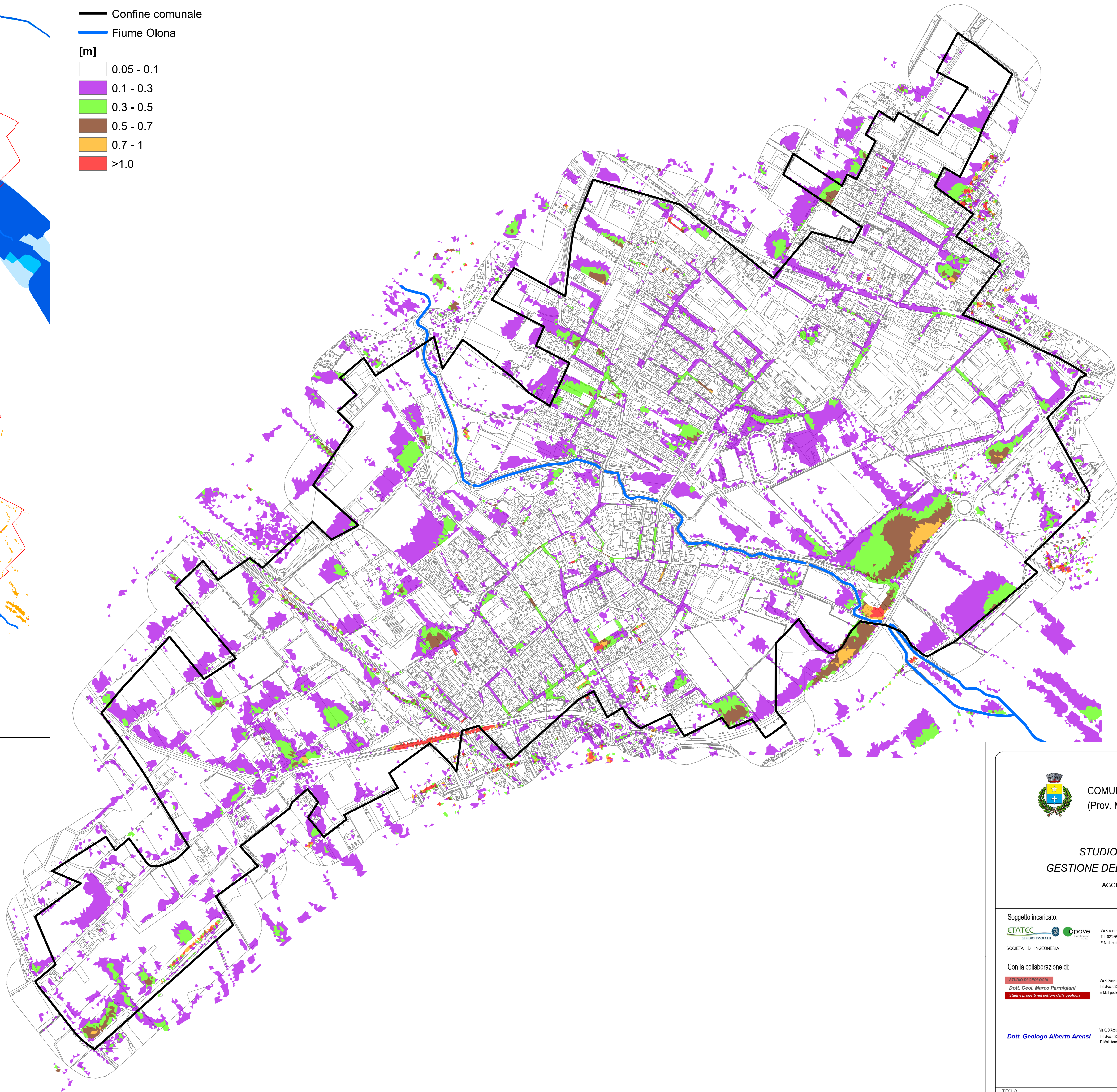
Portata di progetto T=100 anni Olona e precipitazione T=100 anni
